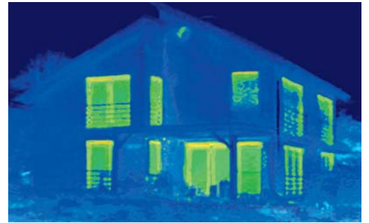
Po fachowo przeprowadzonej wymianie okien na system okienny Schüco Living zdjęcie termograficzne pokazuje znaczący efekt energetyczny takiej inwestycji: pierwotna strata energii została prawie całkowicie zniwelowana
